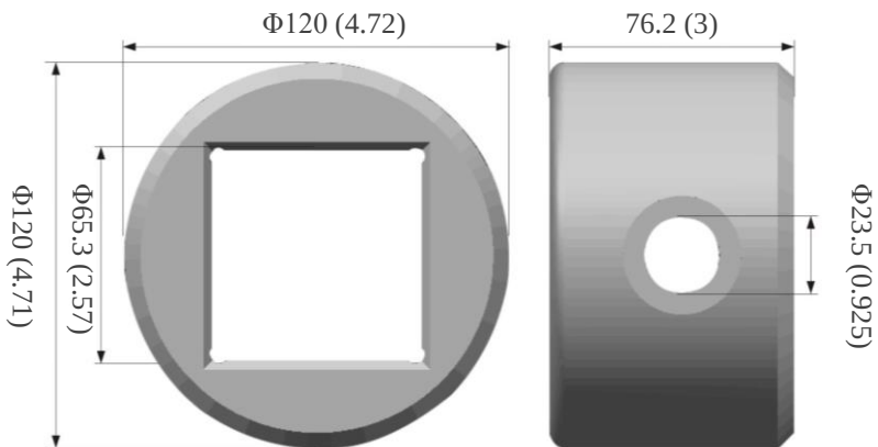
FES/LLH ZPM23 POCKET
